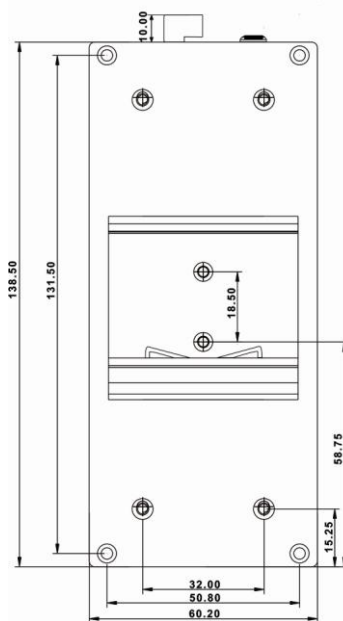
导轨式
