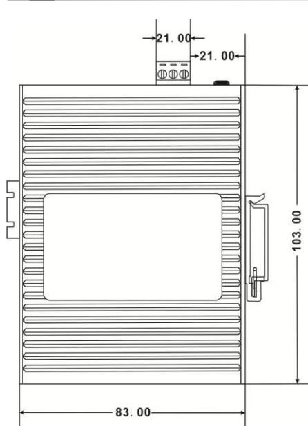
导轨式
