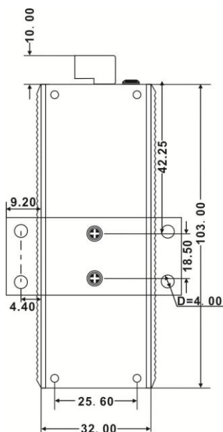
壁挂式2
