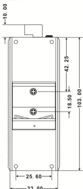
导轨式
