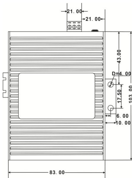
壁挂式1
